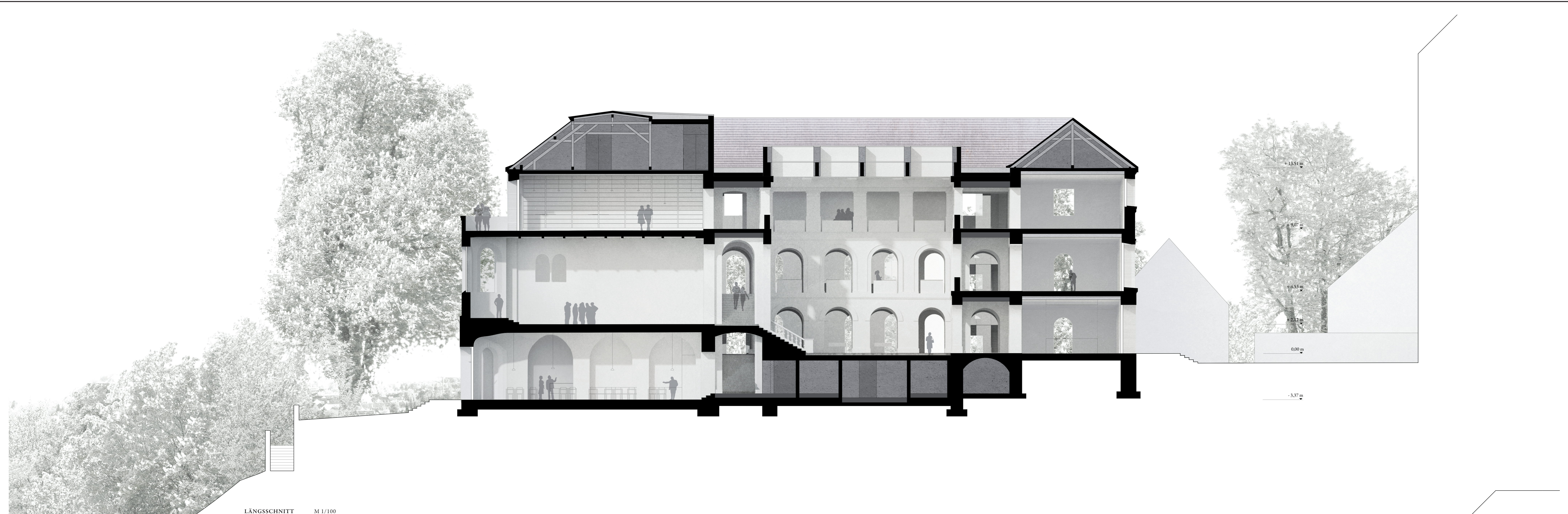
LÄNGSSCHNITT M 1/100
