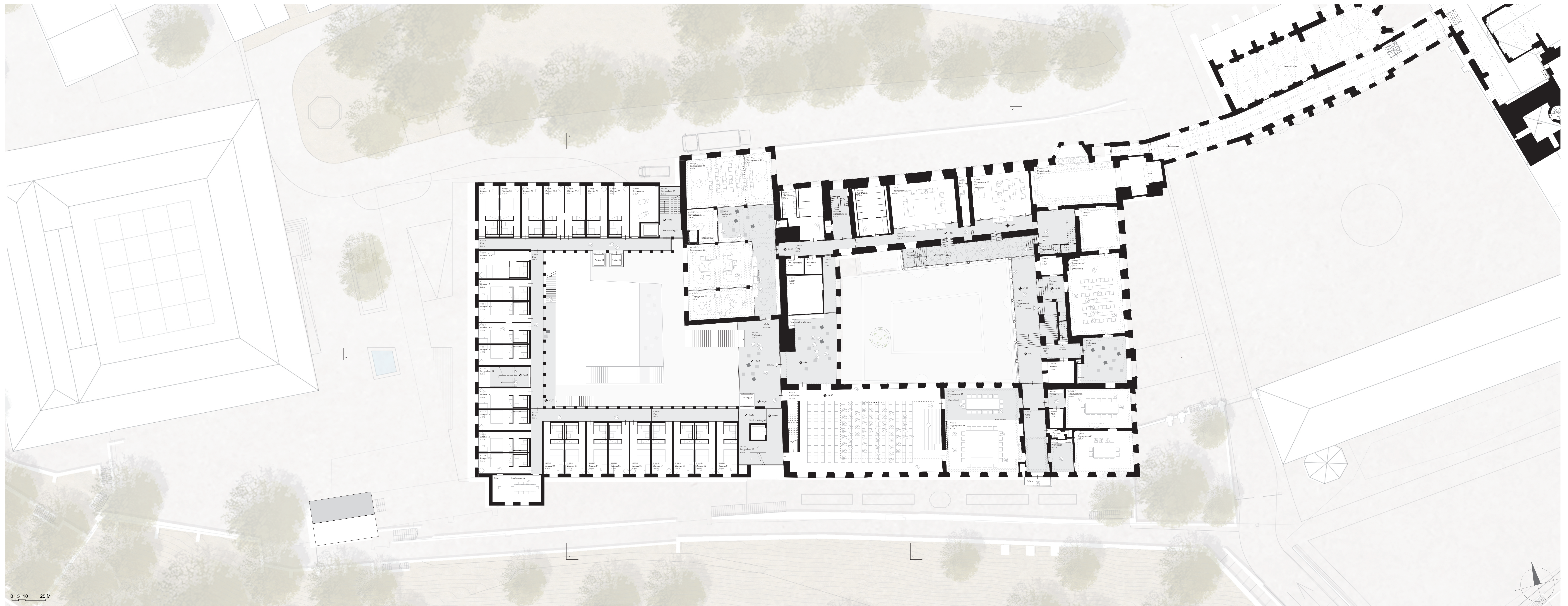
Grundriss 1. Obergeschoss M 1:200
