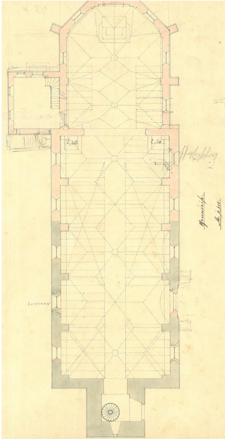
Grundrissplan zur geplanten Erweiterung der Pfarrkirche
