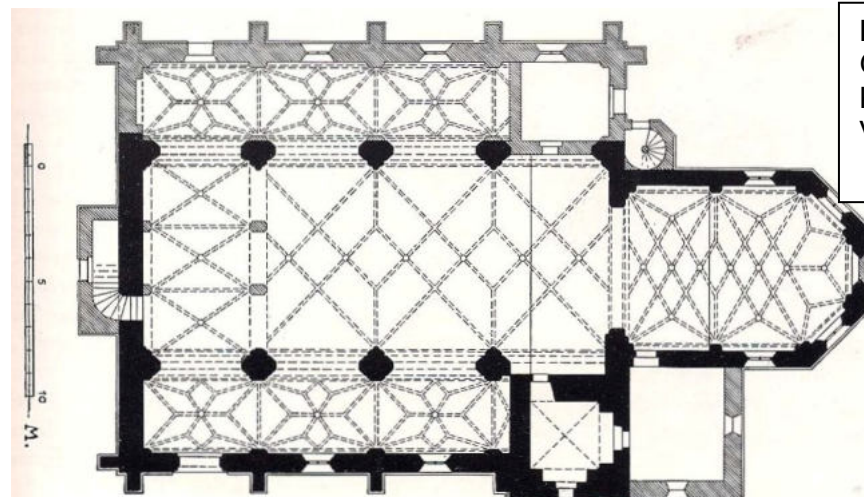
Fig. 45. Feldkirchen. Kirche. Grundriß.
